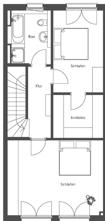
1. Obergeschoss
