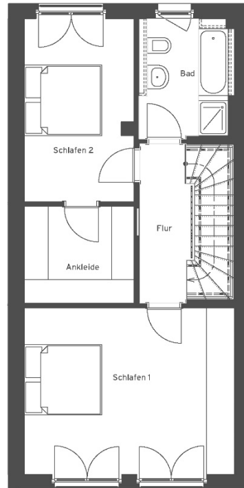
1. Obergeschoss
